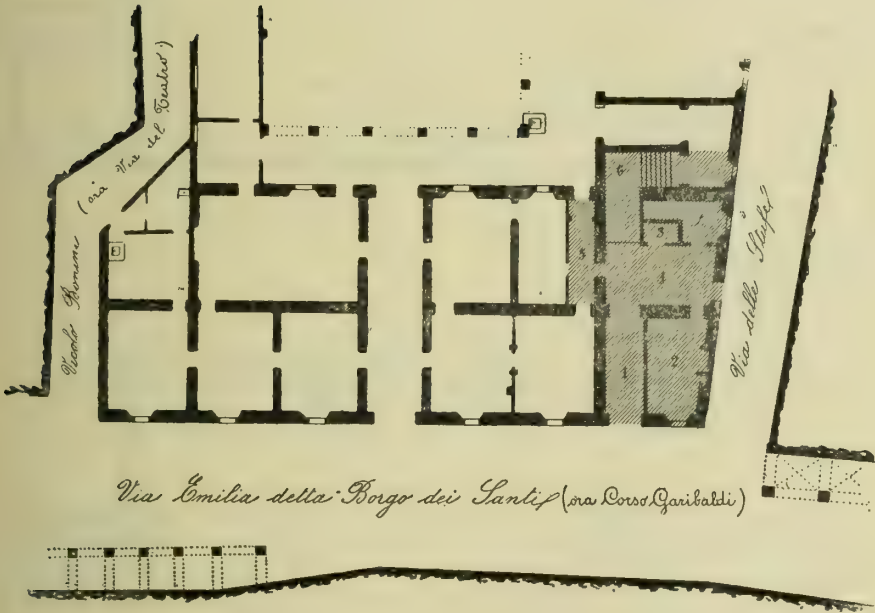
PIANTA DI UNA PARTE DEL PIANTERRENO.
